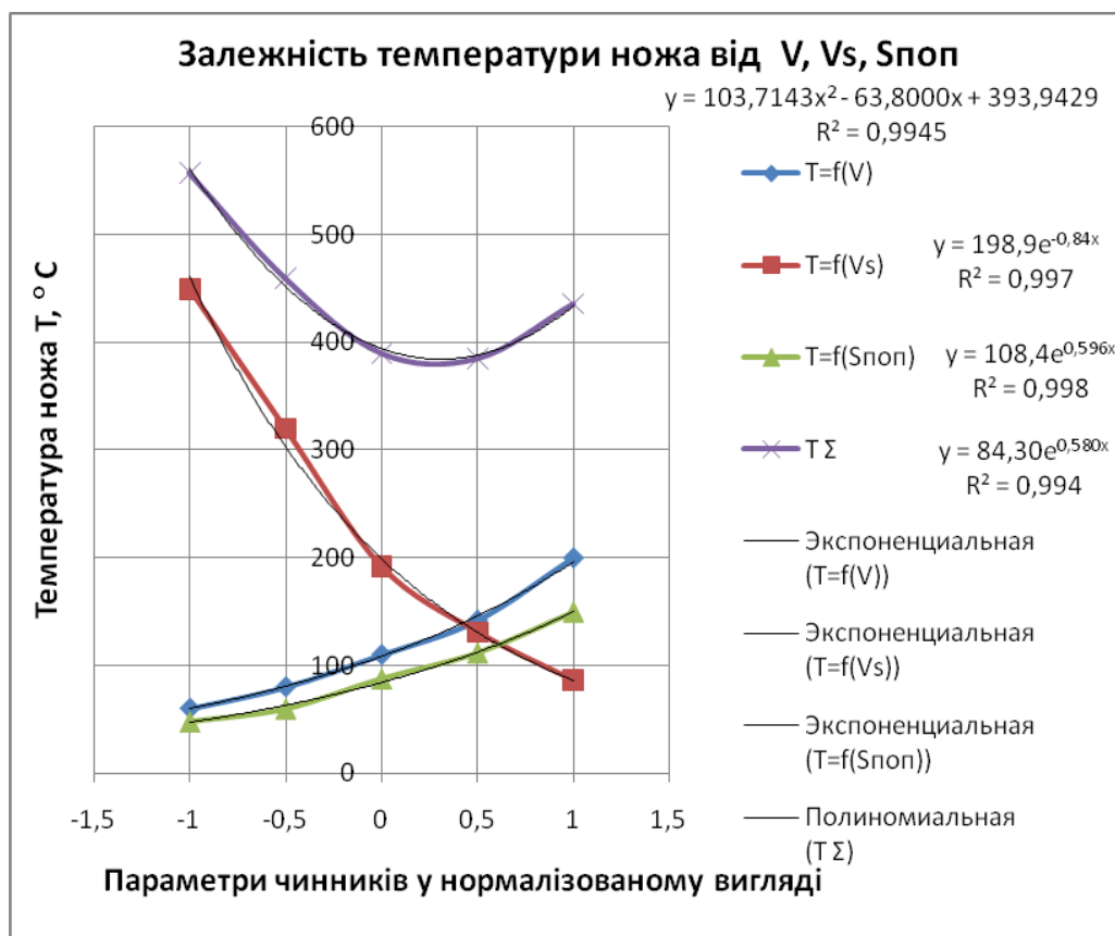
Рис. 1. Залежність температури ножа від швидкості різання, швидкості подачі і подачі на врізання у системі нормалізованих координат
