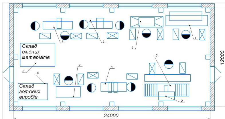
Рис. 6. Планування цеху зі створення фасаду №1 Рамка-скло
