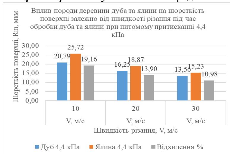
Рис. 2. Порівняння шорсткості поверхні дуба та ялини від швидкості різання
