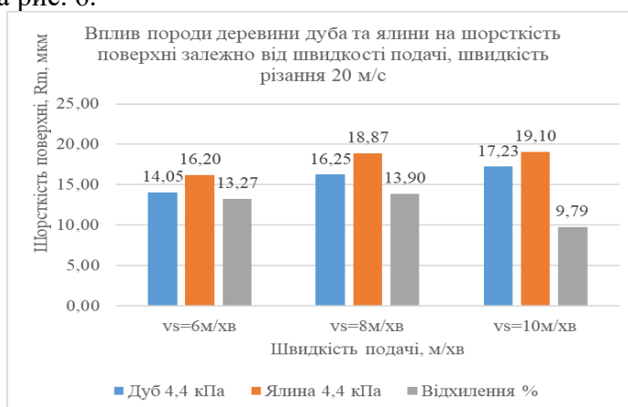
Рис. 6. Порівняння шорсткості поверхні дуба та ялини від швидкості подачі
