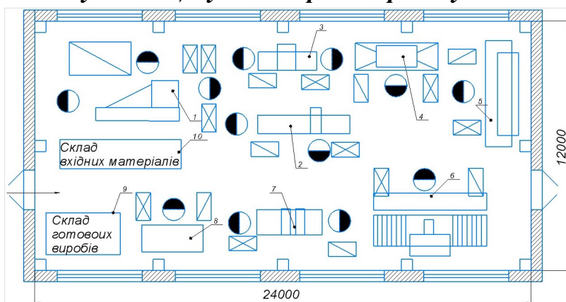
Рис. 7. Планування цеху зі створення фасаду №2 Рамка-тахля
