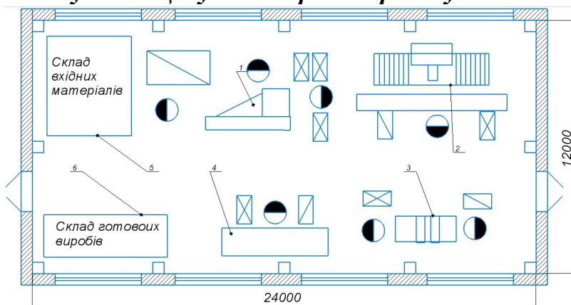
Рис. 8. Планування цеху зі створення фасаду №3 МЩ
