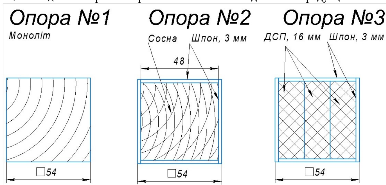
Рис. 3. Три види перерізів опорних елементів різних конструкцій
