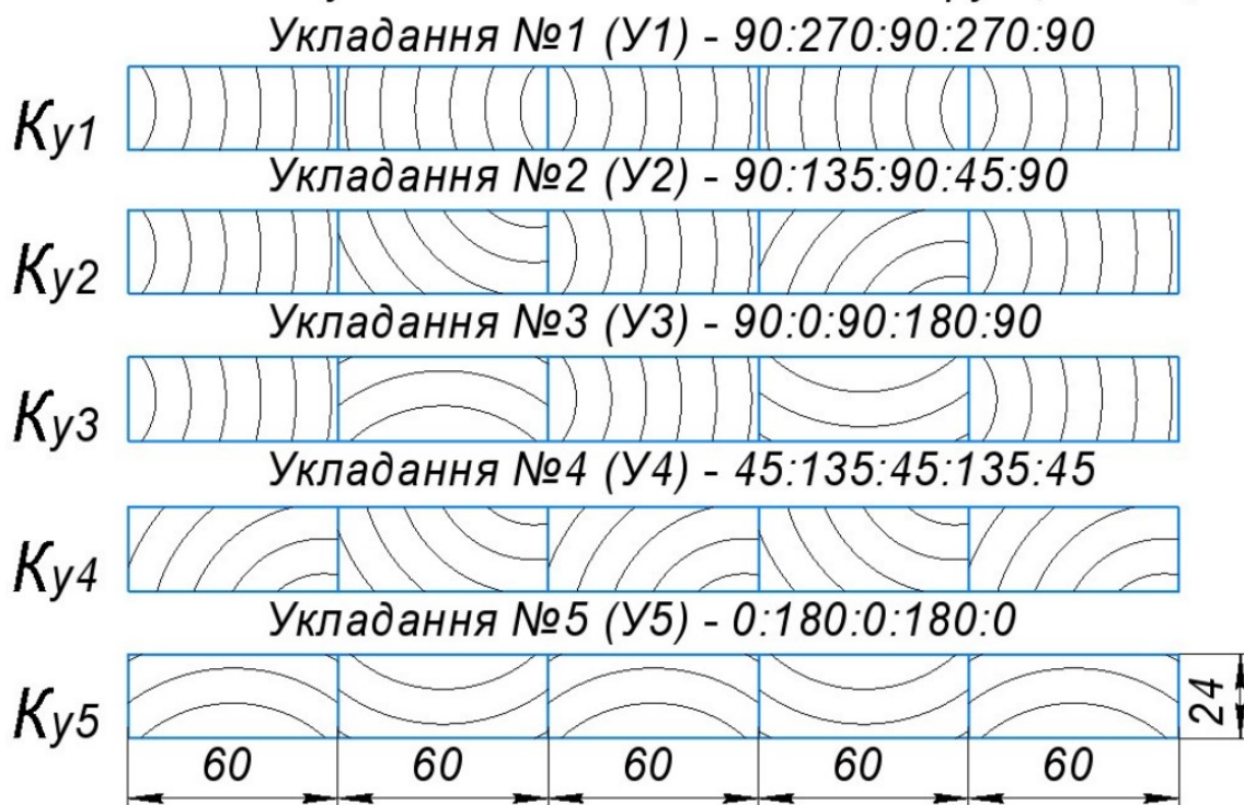
Рис. 3. Конструкції МЩ із деревини бука звичайного ( Fagus sylvatica L.) за способом укладання рейок
