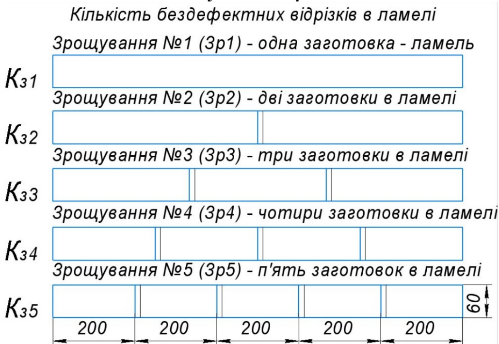
Рис. 4. Різновиди ламелей із бездефектних відрізків деревини в конструкціях МЩ із деревини бука звичайного ( Fagus sylvatica L.)
