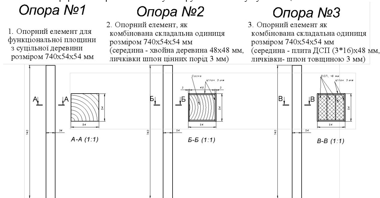
Рис. 2. Три види опорних елементів для дослідження
