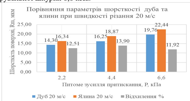
Рис. 4. Порівняння шорсткості поверхні дуба та ялини від притискання
