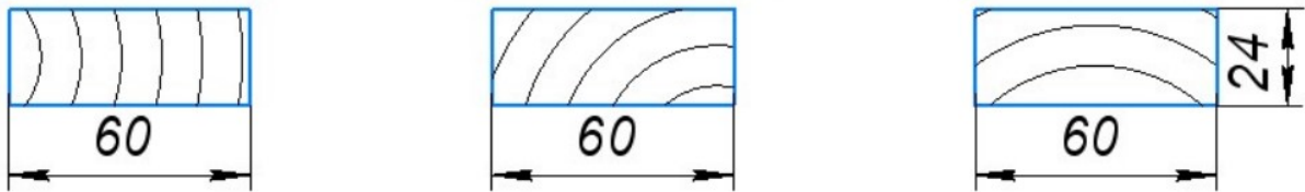
Рис. 2. Види поперечних перерізів рейок за кутами нахилу річних кілець до пластів (радіальний – 61-90^\circ ; напіврадіальний – 31-60^\circ ; тангентальний – 1-30^\circ )
